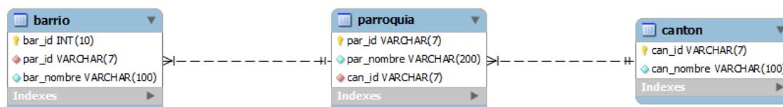
Diagrama entidad - relación
